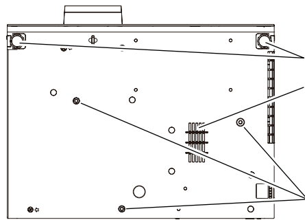
Места расположения регулируемых ножек и отверстий под винты для потолочного крепления
